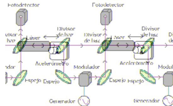
Fig. 6 Interferómetro láser heterodino tipo Mach-Zehnder.
