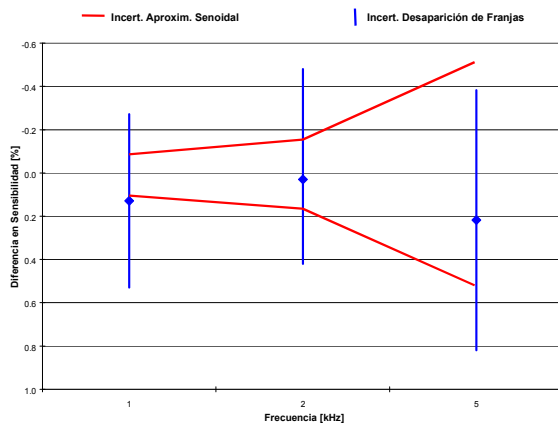
Fig. 8 Calibración de un acelerómetro patrón.
