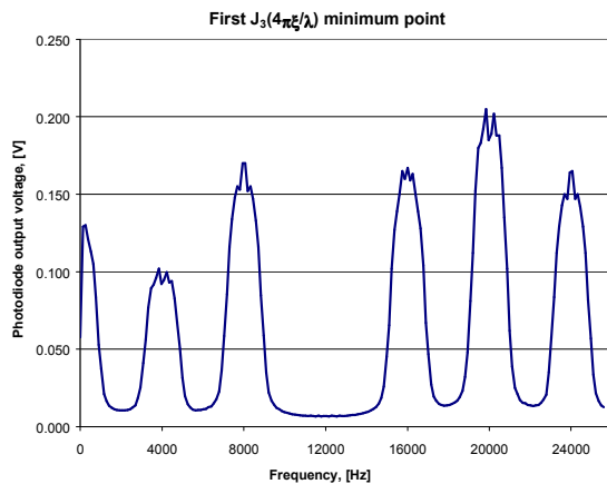
Fig. 3 Espectro de la señal de salida cuando el espejo se mueve a 4 kHz con x=321 nm.
