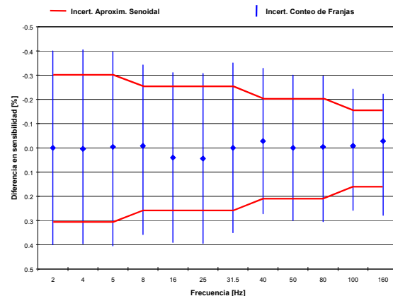
Fig. 7 Calibración de un vibrómetro láser.
