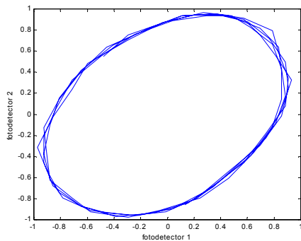
Fig. 5 Señales de salida de las dos unidades de detección de un interferómetro en cuadratura.
